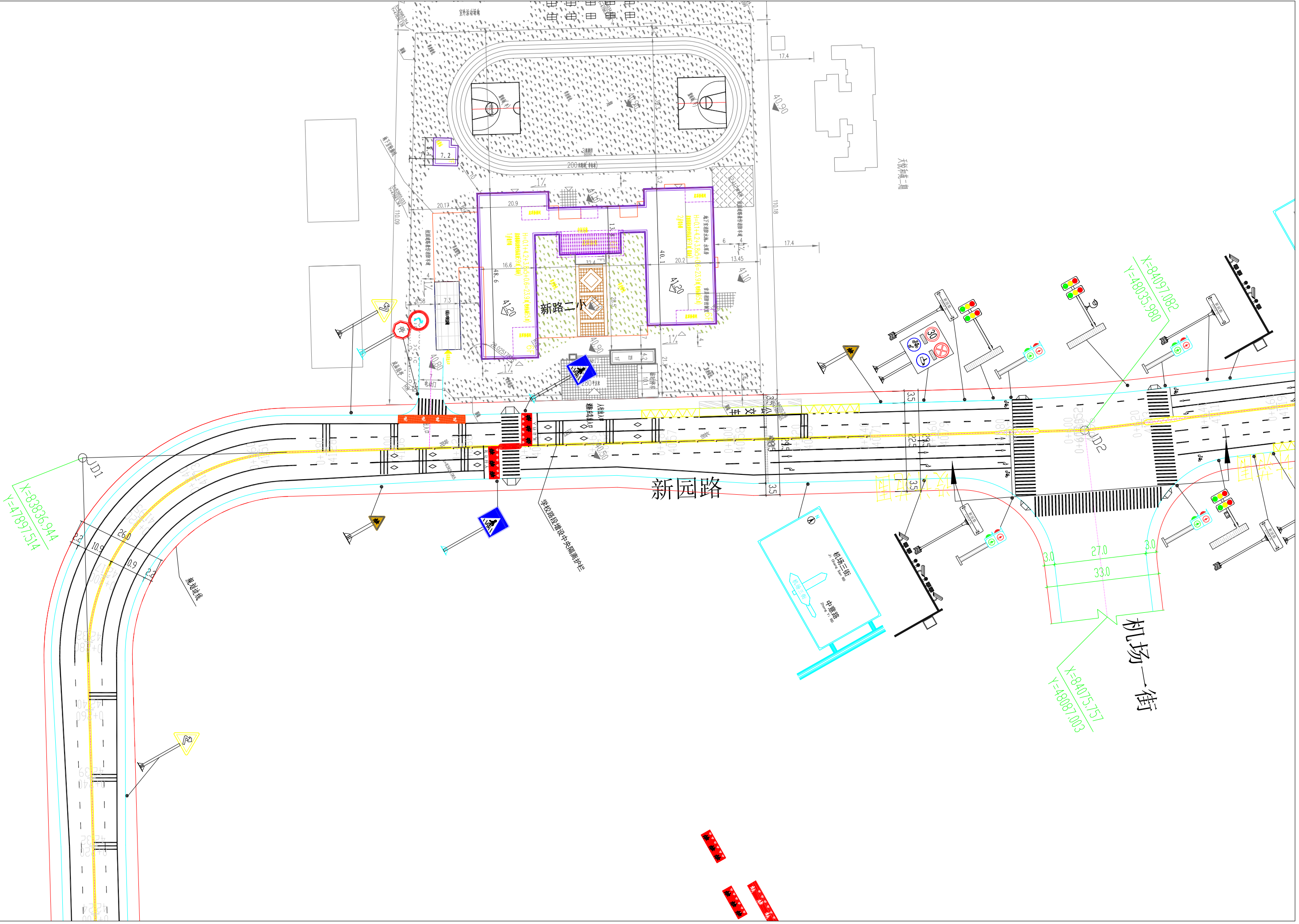
交通设施平面图
